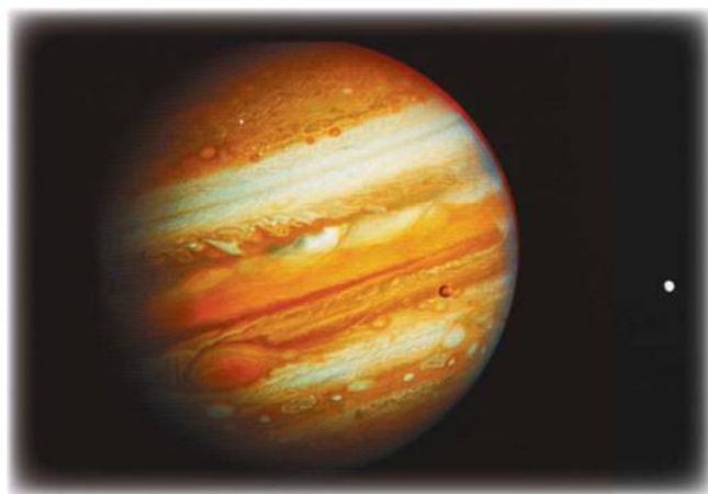
↑ Вид Юпитера в телескоп. Яркая точка справа — один из спутников этой планеты
