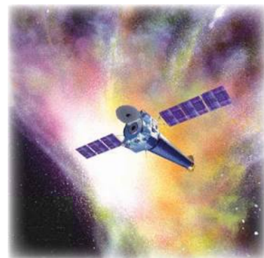
Рентгеновский телескоп в космосе
