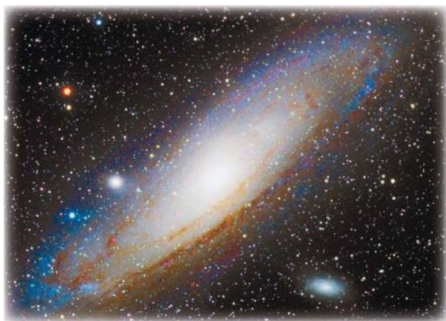
Туманность Андромеды и два ее спутника: эллиптическая галактика М 32 и сфероидальная система М 110
