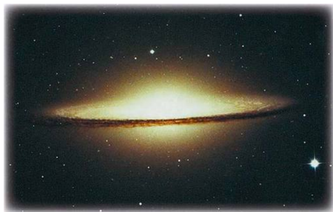
† Ядро галактики Сомбреро (M 104) в созвездии Дева светится очень ярко
