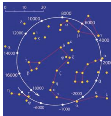
Северный полюс мира был у \tau Геркулеса, \alpha Дракона, сейчас он возле \alpha Малой Медведицы, а затем будет у \gamma Цефея
