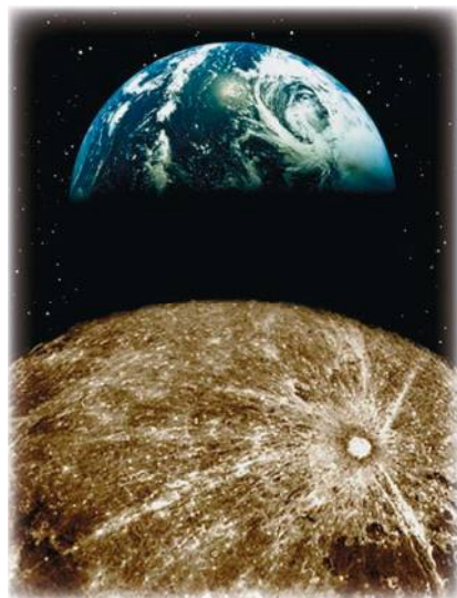
Фотография Земли, сделанная космическим аппаратом со стороны Луны
