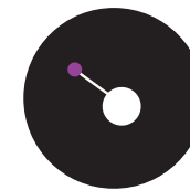
δ Геркулеса
