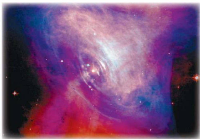
↑ В центре Крабовидной туманности — пульсар, видный в оптическом диапазоне
