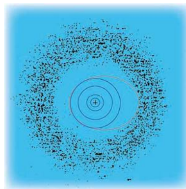
Схема расположения пояса Койпера (35—50 тыс. а. е. от Солнца)
