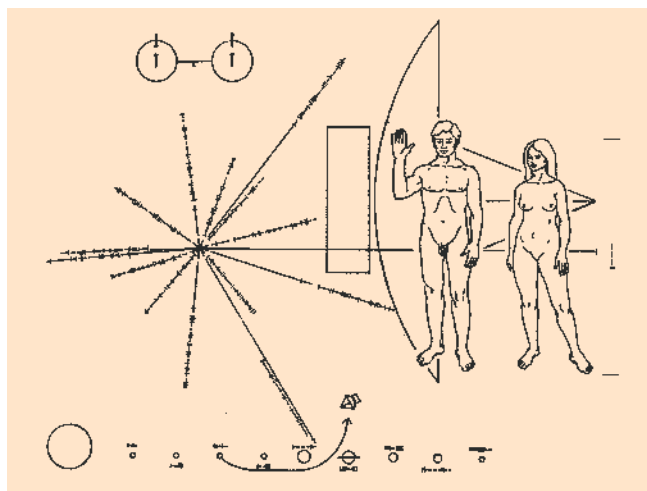
↑ Такое послание было отправлено в космос вместе с аппаратом «Пионер-10»
