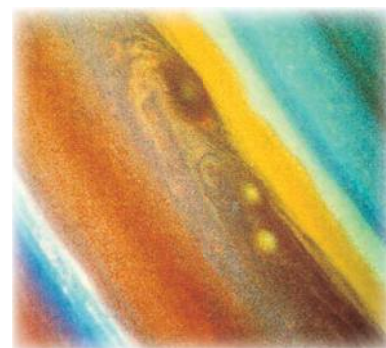
Фрагмент снимка поверхности Сатурна
